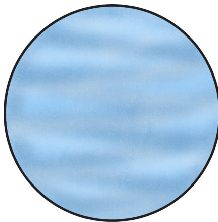
Uranus
