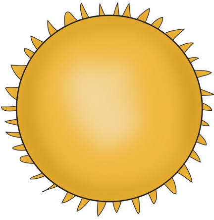
sun
