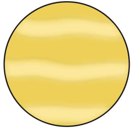
Venus
