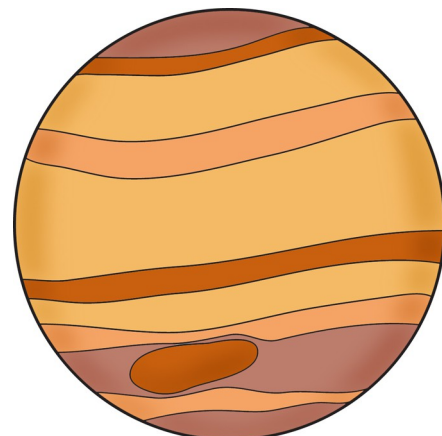
Jupiter
