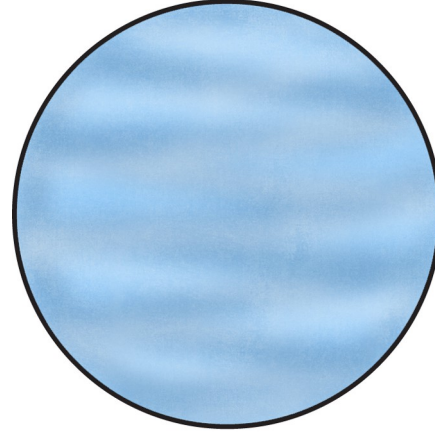
Uranus
