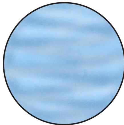
Uranus
