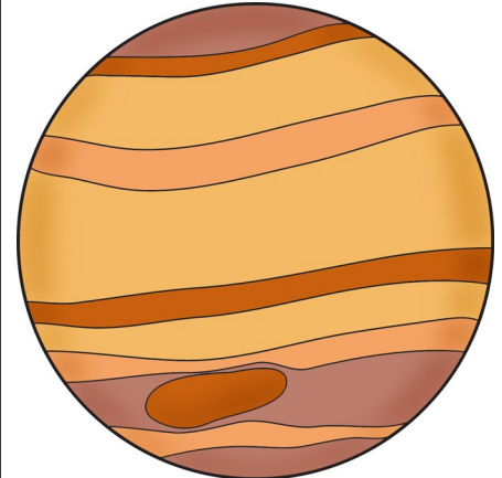
Jupiter
