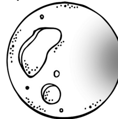
penumbral
