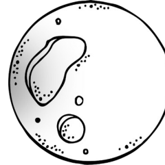
penumbral
