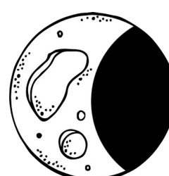
penumbral
